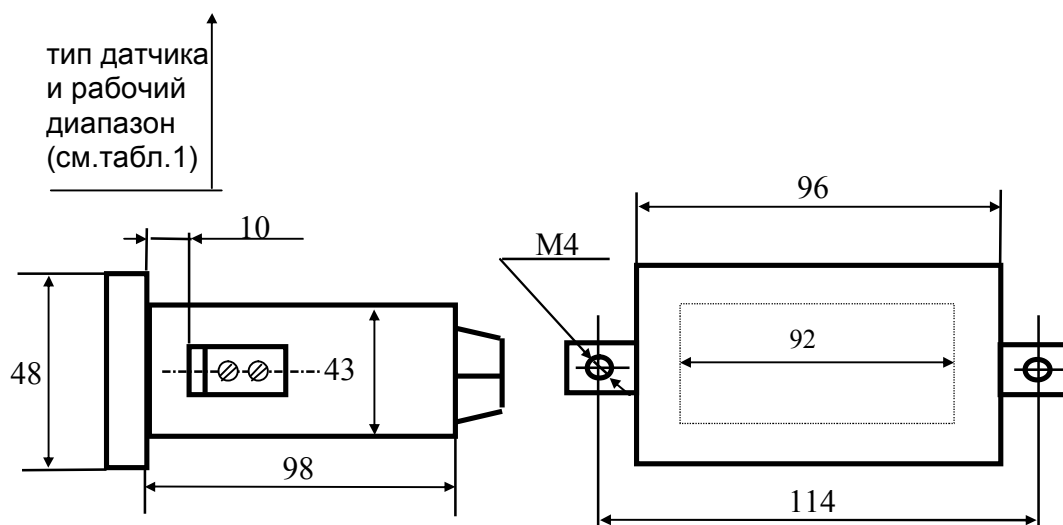
Рис. 1а Габаритные размеры
